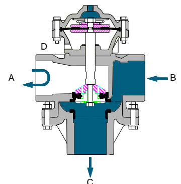
Backflush mode
